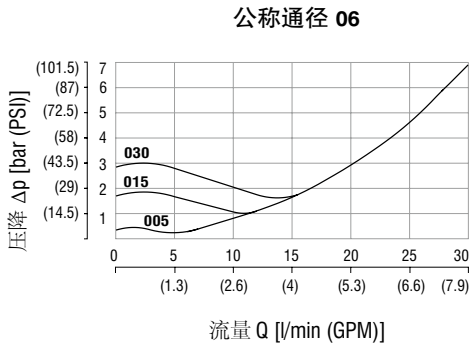
压降Δp - 流量曲线
